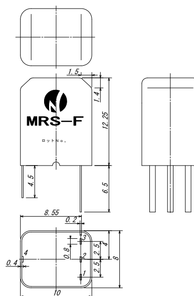
外形図
